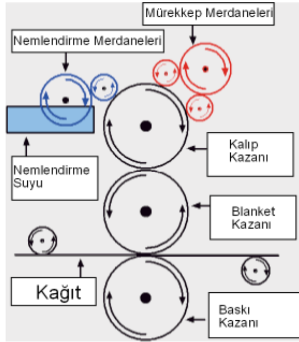
Şekil 8.9. Ofset Baskı tekniği
