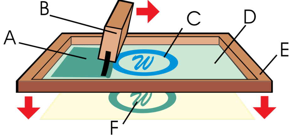
Şekil 8.10. A. Mürekkep. B. Çekçek. C. Görüntü. D. İpek kumaşa foto emülsiyon. E. Çerçeve. F. Basılan görüntü.
